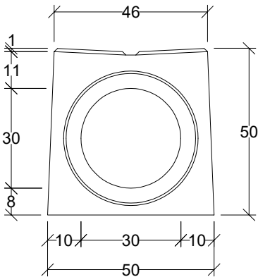
Widok gniazdo
