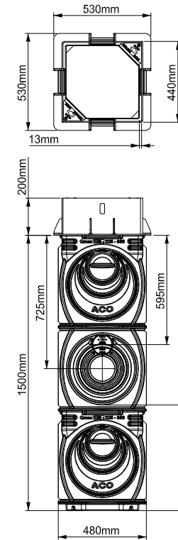
32978 Studzienka odpływowa z osadnikiem z pokrywą ze stali ocynkowanej D400
