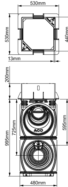
32977 Studzienka odpływowa z pokrywą ze stali ocynkowanej D400
