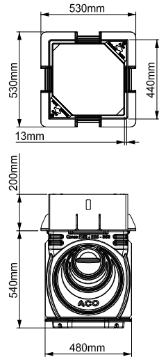
32976 Studzienka rewizyjna z pokrywą ze stali ocynkowanej D400
