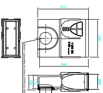
Jednozęściowa skrzynka odpływowa z koszem osadczym
