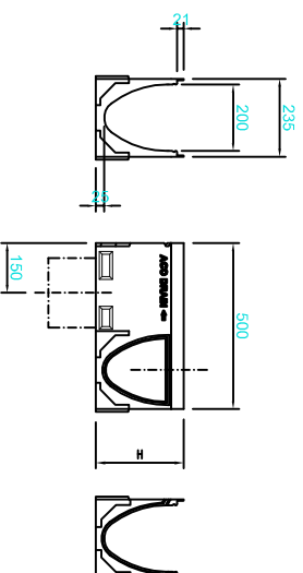
Korytka o długości 0,5m z przetłoczeniami: w ściankach - do połączeń "T" i "I" w dnie - do rury Ø200
