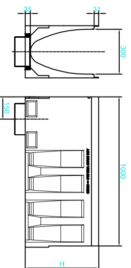
Korytka o długości 1m z otworami i uszczelką do rury Ø200
